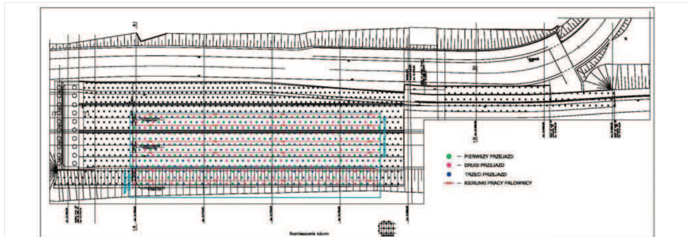
Rys. 2. Plan palowania – ETAP III
